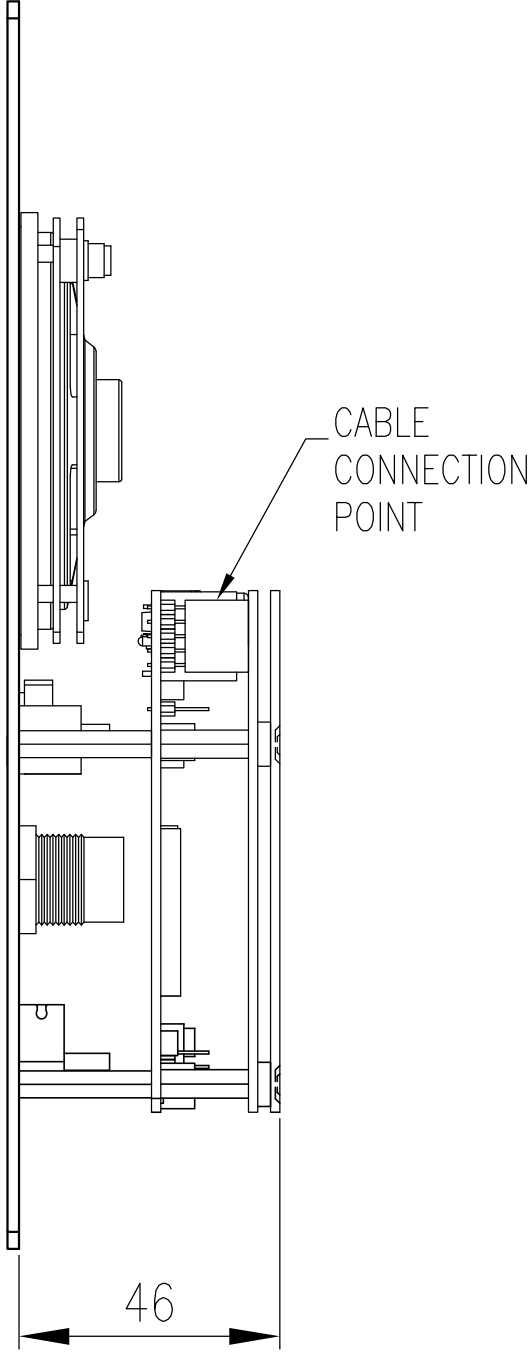
VSL-391-LR
